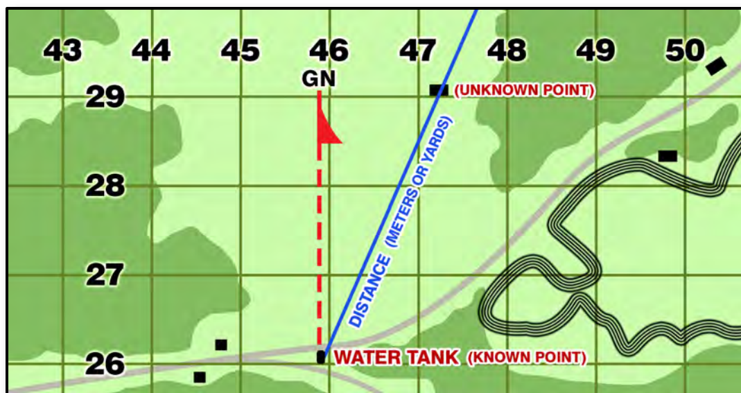
Using Polar Coordinates
